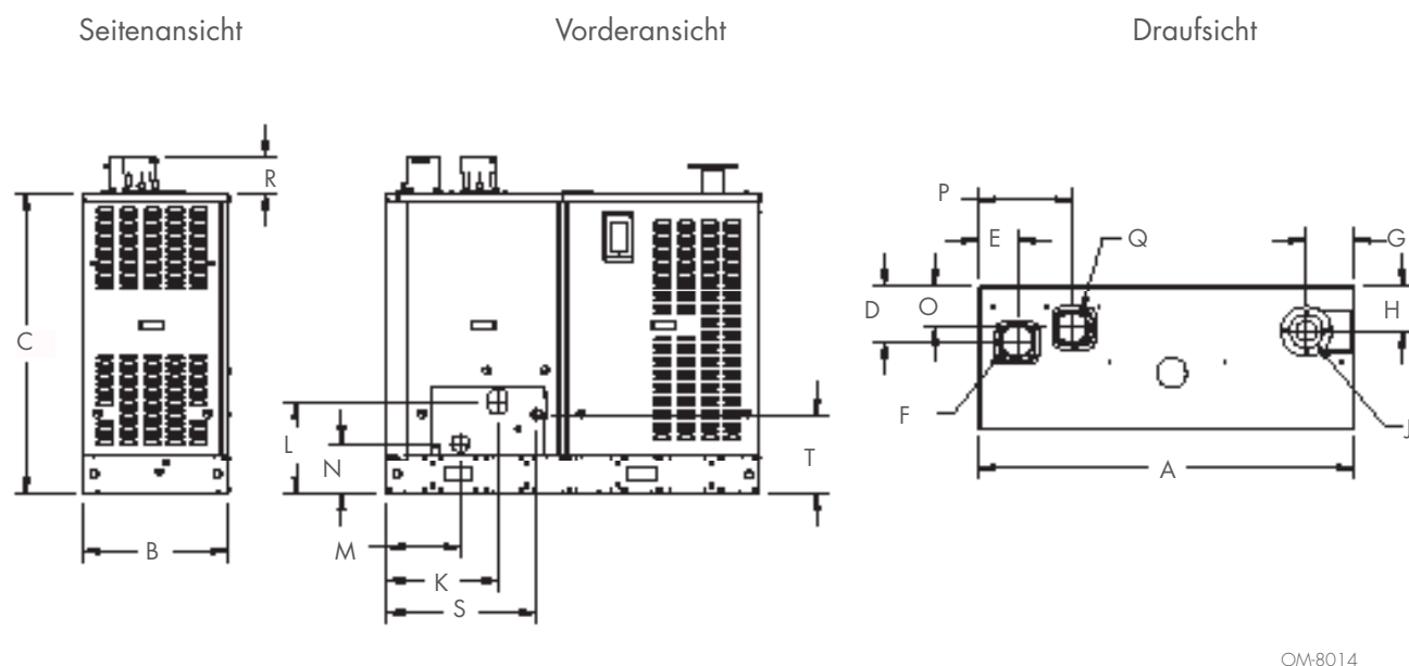
ABBILDUNG 8-2: LX MODELLE 200 - 300 GERÄTEABMESSUNGEN FÜR DEN INNENBEREICH
