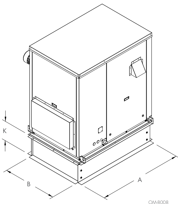
ABBILDUNG 12-1: GEHÄUSE FÜR DEN AUSSENBEREICH AUF SOCKEL
