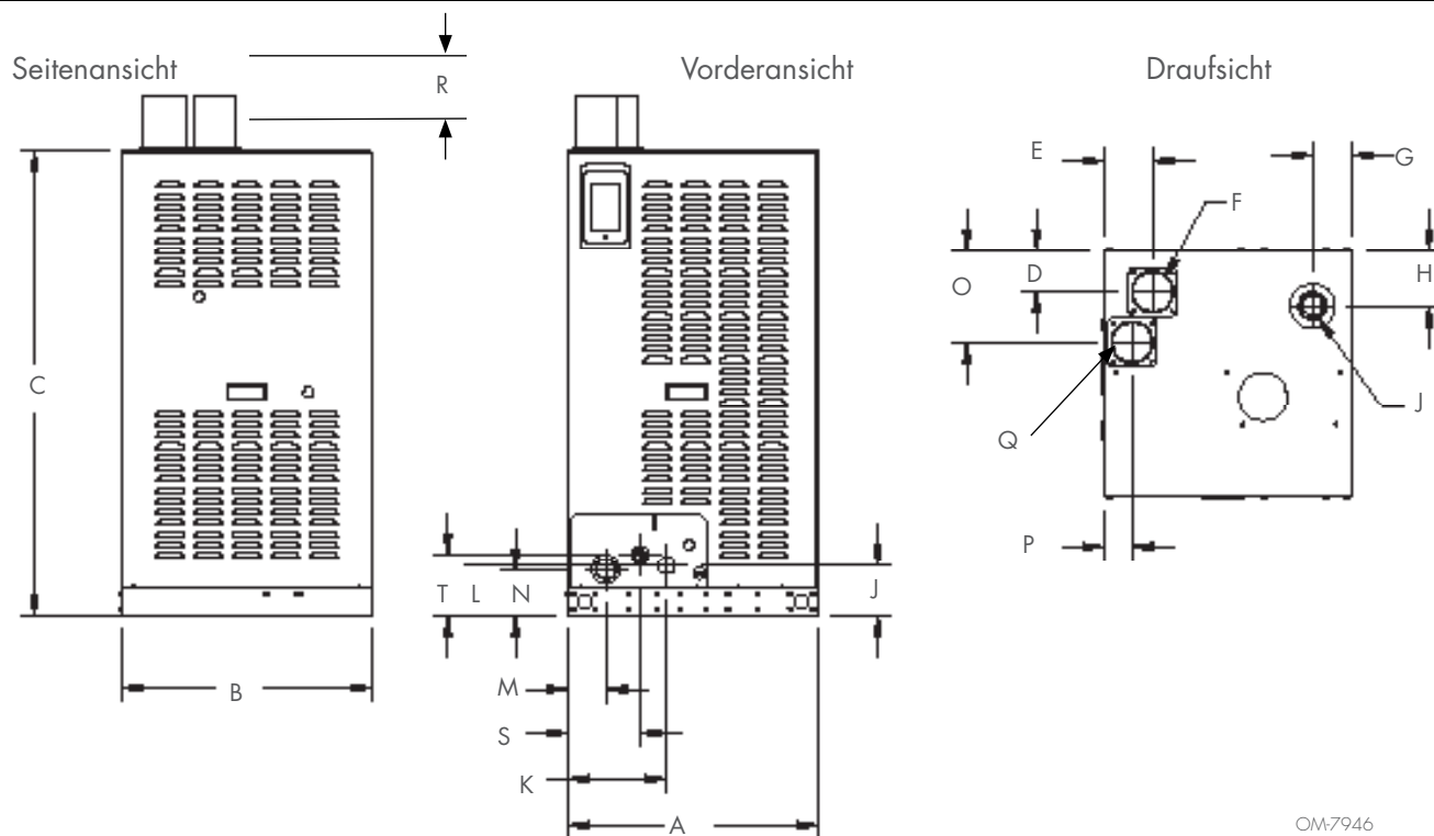
ABBILDUNG 8-1: LX MODELLE 50 - 150 GERÄTEABMESSUNGEN FÜR DEN INNENBEREICH
