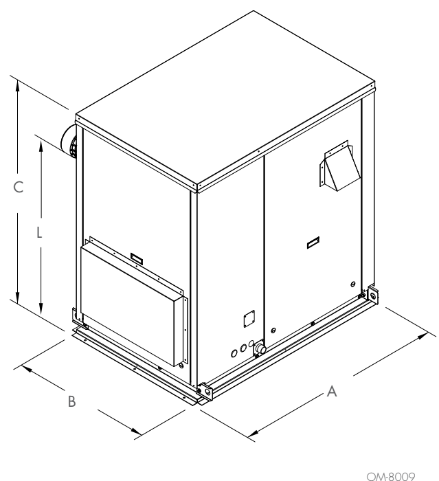
ABBILDUNG 12-2: GEHÄUSE FÜR DEN AUSSENBEREICH EBENERDIG MONTIERT
