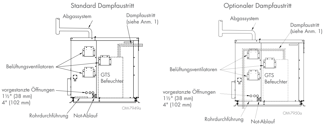
ZEICHNUNG 12-1: GTS – LX BEFEUCHTER GEHÄUSE ZUR AUSSENAUFSTELLUNG MIT STANDARD- ODER INTERNEM DAMPFAUSTRITT
