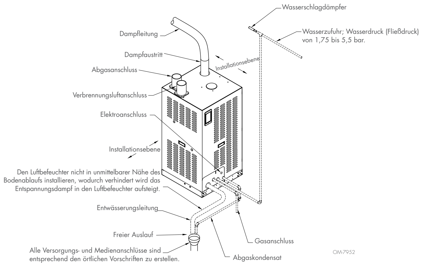
ZEICHNUNG 14-1: GTS - LX BEFEUCHTER ÜBERSICHT DER VERROHRUNG
