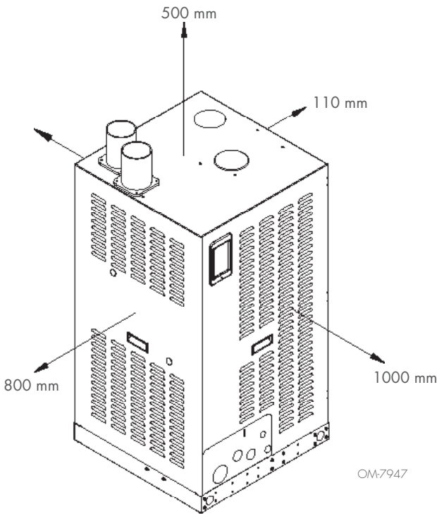
ZEICHNUNG 10-2: GTS - LX BEFEUCHTER MINDESTABSTÄNDE
