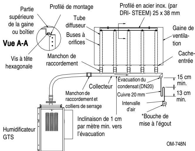
Figure 21-2 : Unité Rapid-SORB Collecteur sous la gaine
