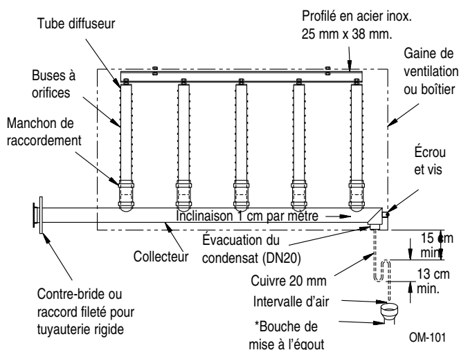
Figure 21-1: UNITÉ RAPID-SORB Collecteur à l'intérieur de la gaine
