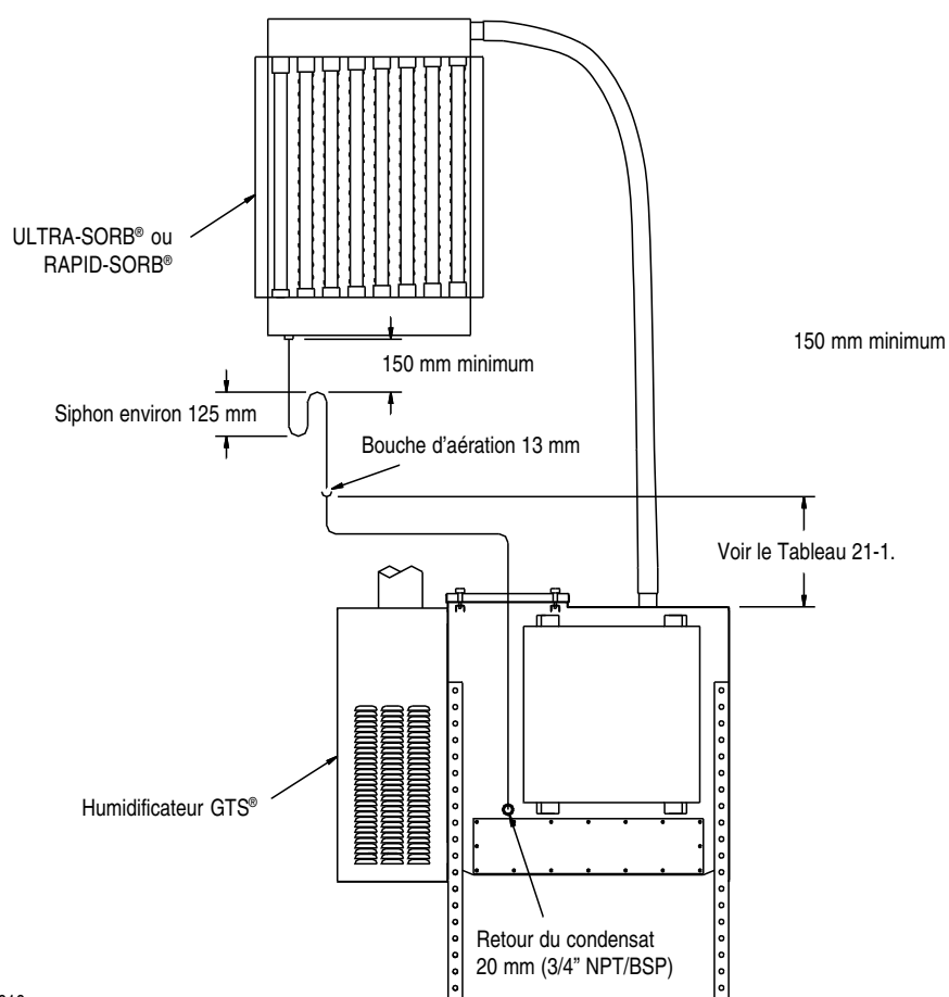
Figure 20-1 : Retour de condensat à l'humidificateur
