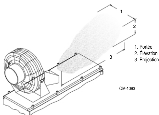
Figure 23-1 Ventilateur DIFFUSEUR DE ZONE
