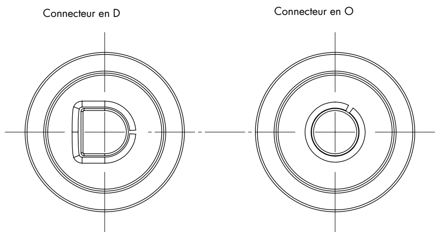
FIGURE 39-1 : CONNECTEURS
