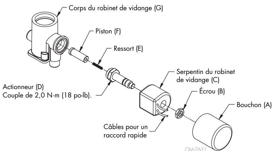
FIGURE 40-2 : MAINTENANCE DU CORPS DU ROBINET DE VIDANGE
