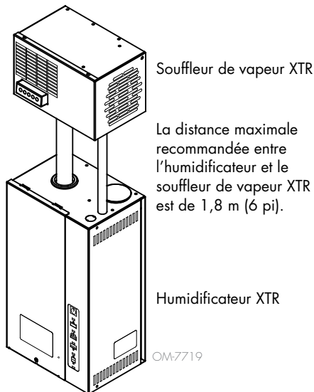
FIGURE 24-1 : DISPERSION DU SOUFFLEUR DE VAPEUR XTR
