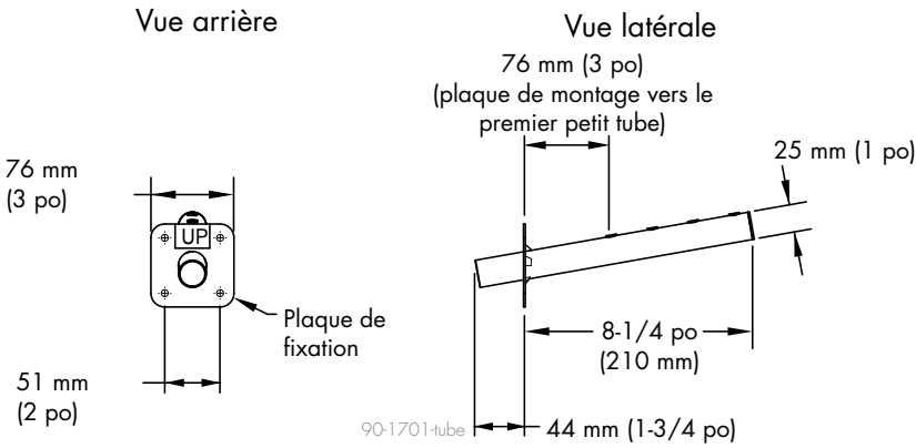
FIGURE 23-1 : DIMENSIONS DU TUBE DE DISPERSION XTR
