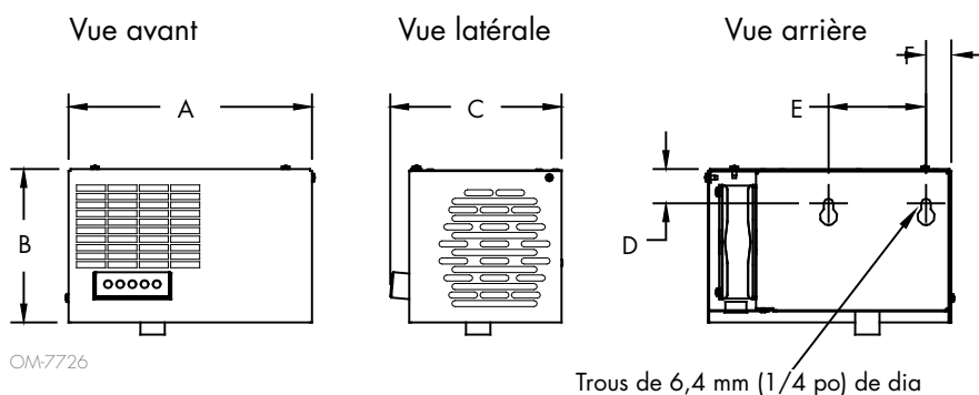
FIGURE 26-1 : DIMENSIONS DU SOUFFLEUR DE VAPEUR XTR
