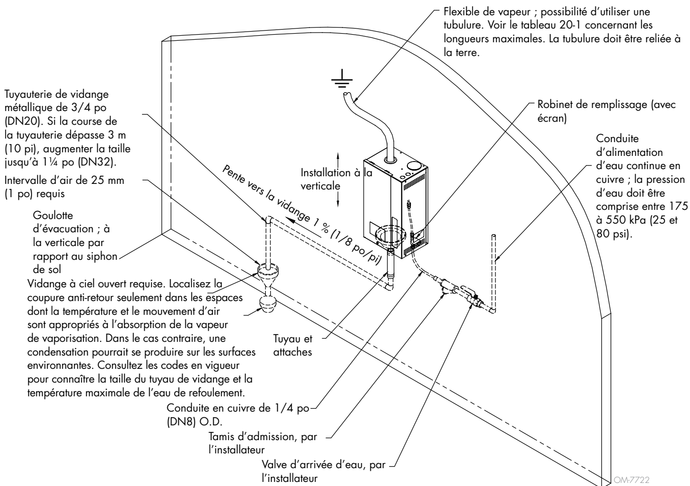
FIGURE 10-1 : VUE D'ENSEMBLE DE LA TUYAUTERIE SUR SITE DE L'HUMIDIFICATEUR XTR
