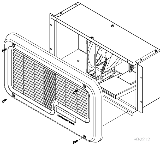
FIGURE 31-1 : MONTAGE DU FAN PACK XTR
