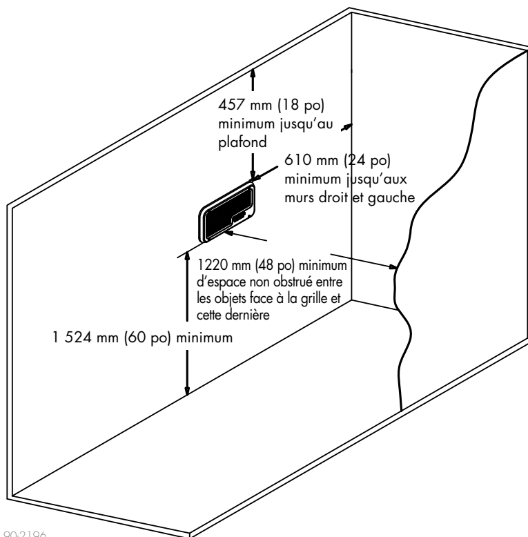
FIGURE 29-1 : DÉGAGEMENTS MINIMUM RECOMMANDÉS AVEC LE FAN PACK XTR DANS L'ESPACE HUMIDIFIÉ
