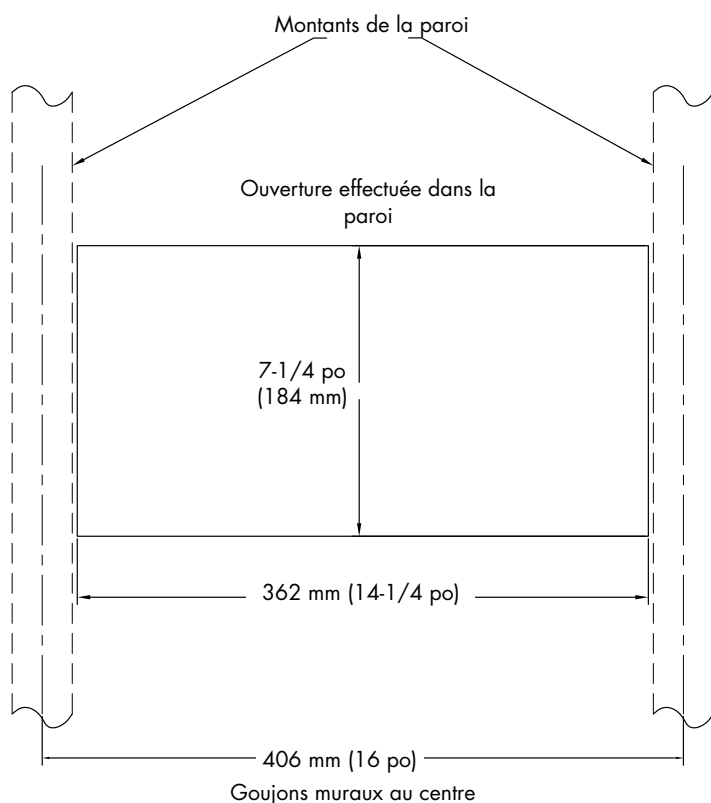
FIGURE 30-2 : DIMENSIONS DES OUVERTURES DE LA PAROI
