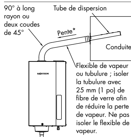
FIGURE 22-1 : TUBE DE DISPERSION XTR MONTÉ PLUS HAUT QUE L'HUMIDIFICATEUR
