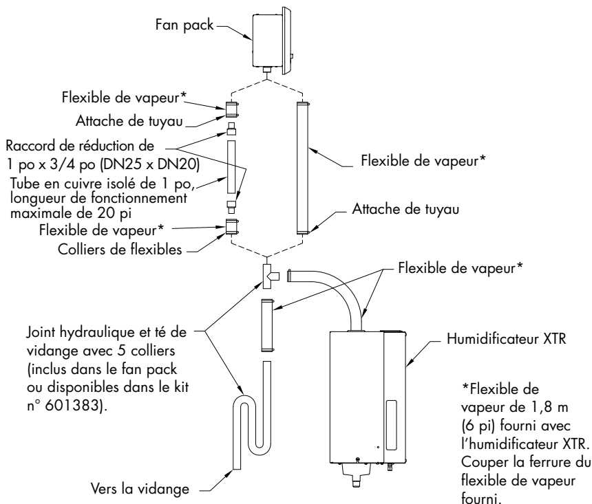
FIGURE 28-2 : RALLONGER LA DISTANCE ENTRE L'HUMIDIFICATEUR ET LE FAN PACK À L'AIDE DU TUYAU EN CUIVRE
