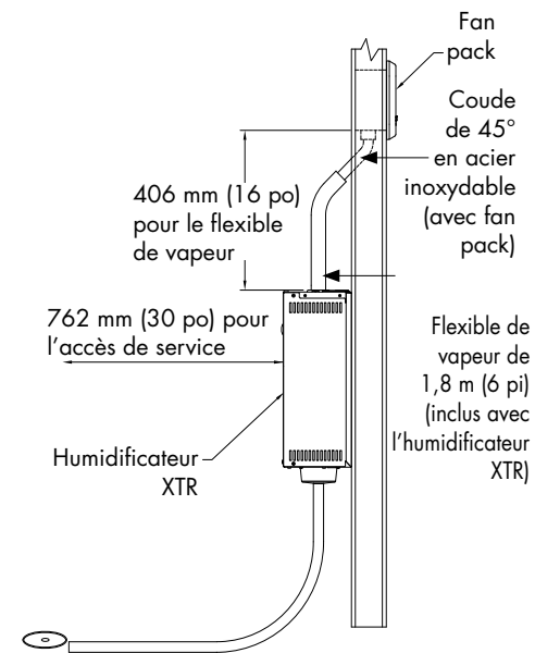
FIGURE 27-1 : DIMENSIONS ET DÉGAGEMENTS RECOMMANDÉS POUR L'HUMIDIFICATEUR ET LE FAN PACK XTR
