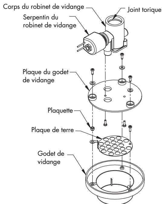
FIGURE 41-1 : MAINTENANCE DE L'ENSEMBLE DE ROBINET DE VIDANGE
