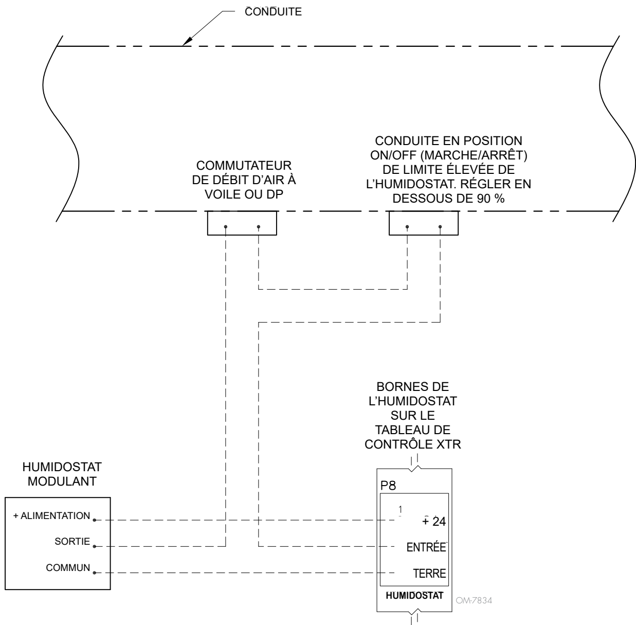
FIGURE 17-1 : CÂBLAGE DE COMMANDE MODULANT TYPIQUE
