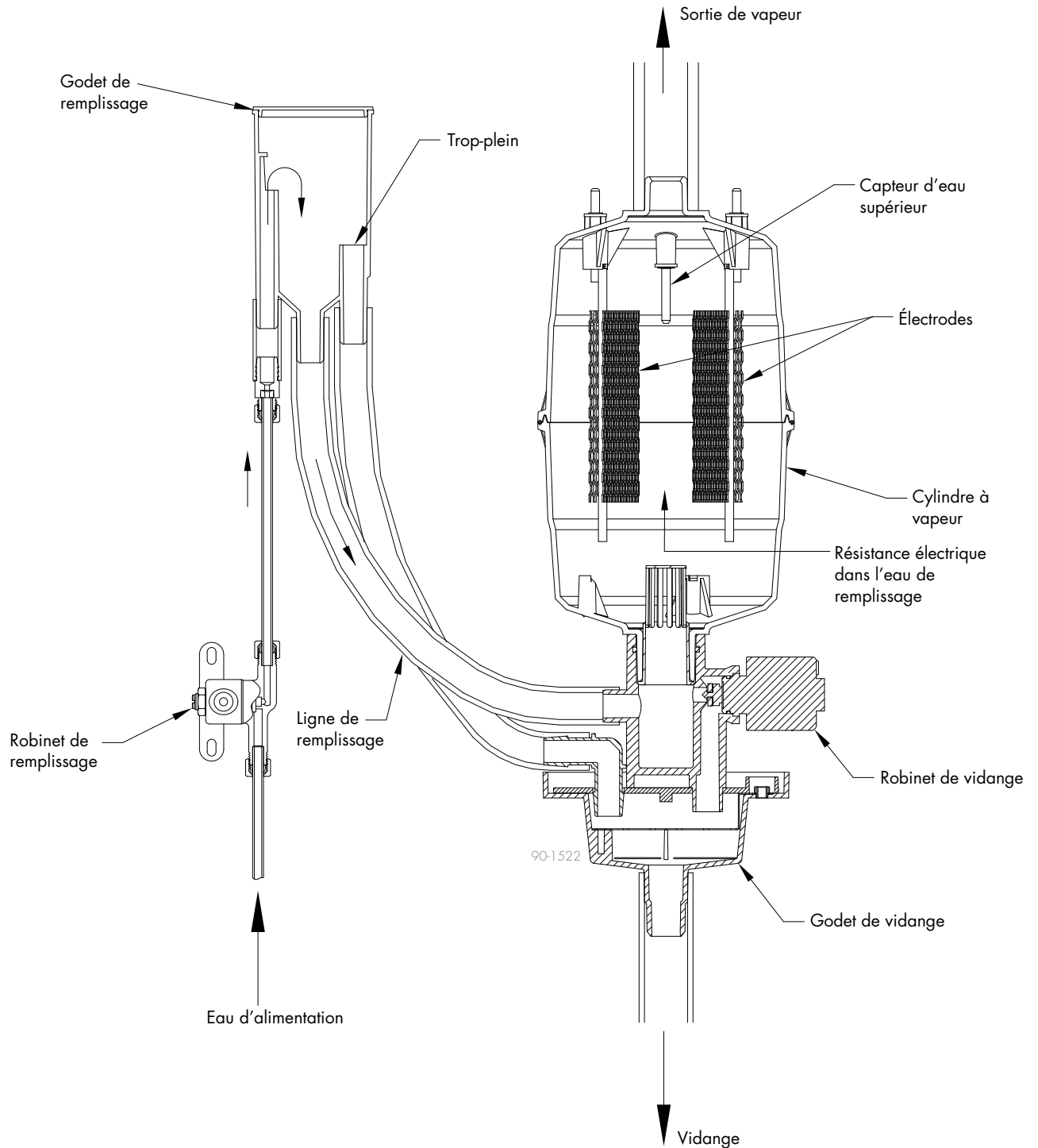
FIGURE 33-1 : PRINCIPE DE FONCTIONNEMENT DE L'HUMIDIFICATEUR XTR
