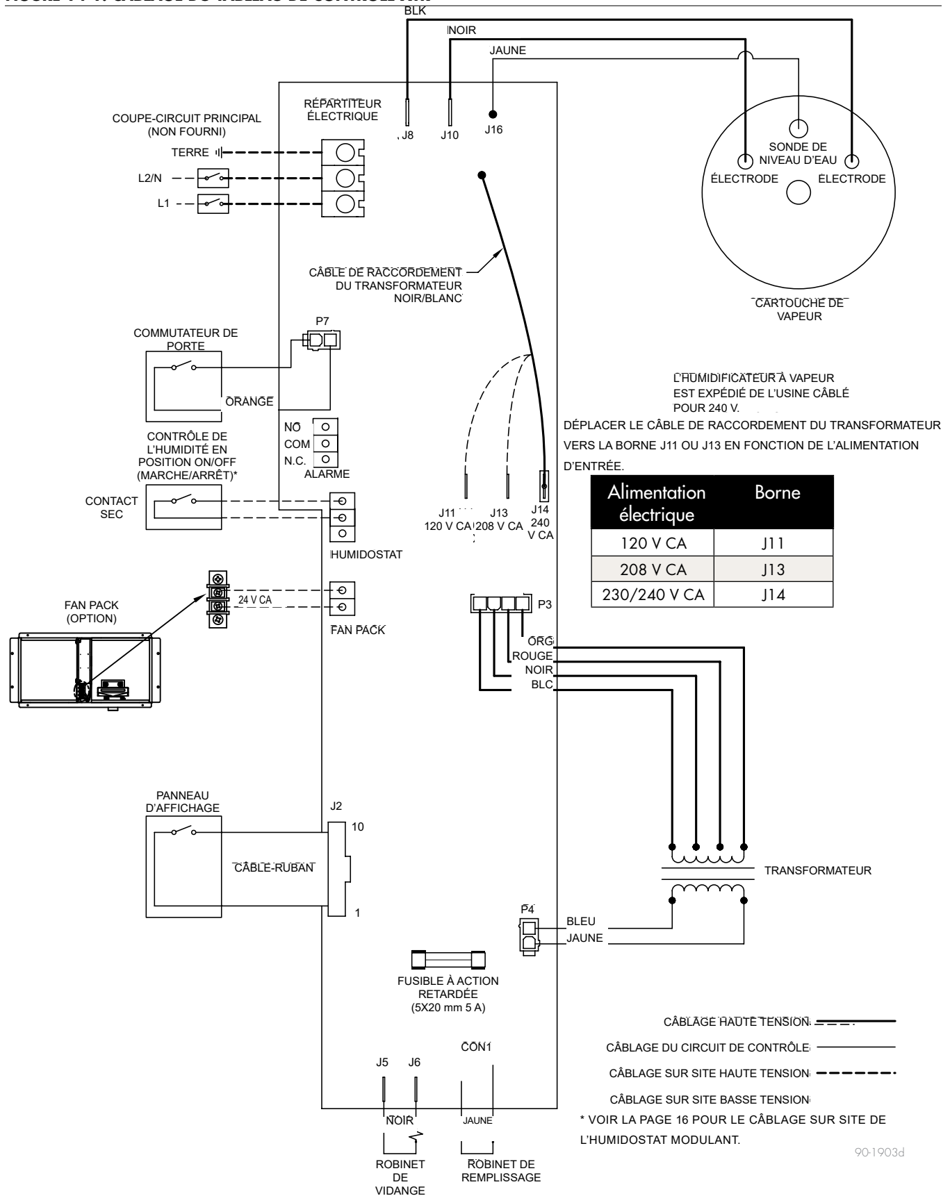
FIGURE 14-1: CÂBLAGE DU TABLEAU DE CONTRÔLE XTR
