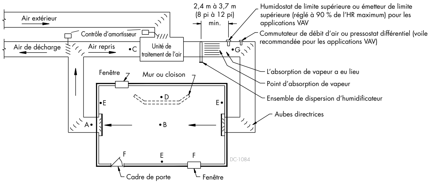
FIGURE 19-1 : EMBLEMES DE CAPTEUR RECOMMANDÉS
