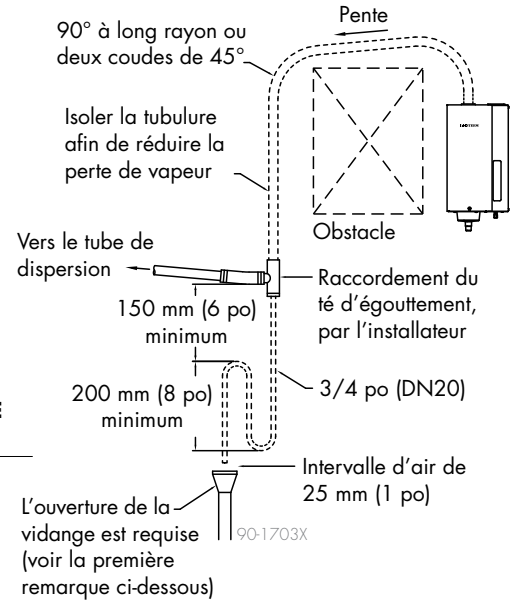
FIGURE 23-3 : RALLONGER LA DISTANCE ENTRE L'HUMIDIFICATEUR ET LE TUBE DE DISPERSION À L'AIDE DU TUYAU EN CUIVRE
