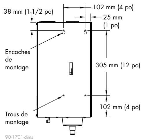
FIGURE 8-1 : TROUS DE MONTAGE DE L'HUMIDIFICATEUR XTR
