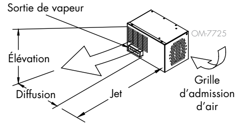
FIGURE 25-1 : ÉLÉVATION, PROPAGATION ET JET DU SOUFFLEUR DE VAPEUR XTR
