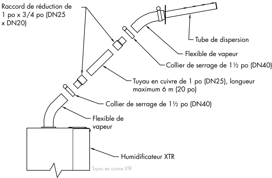
FIGURE 23-3 : RALLONGER LA DISTANCE ENTRE L'HUMIDIFICATEUR ET LE TUBE DE DISPERSION À L'AIDE DU TUYAU EN CUIVRE
