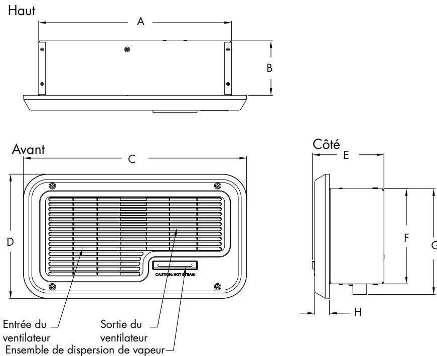
FIGURE 28-1 : DIMENSIONS DU FAN PACK XTR
