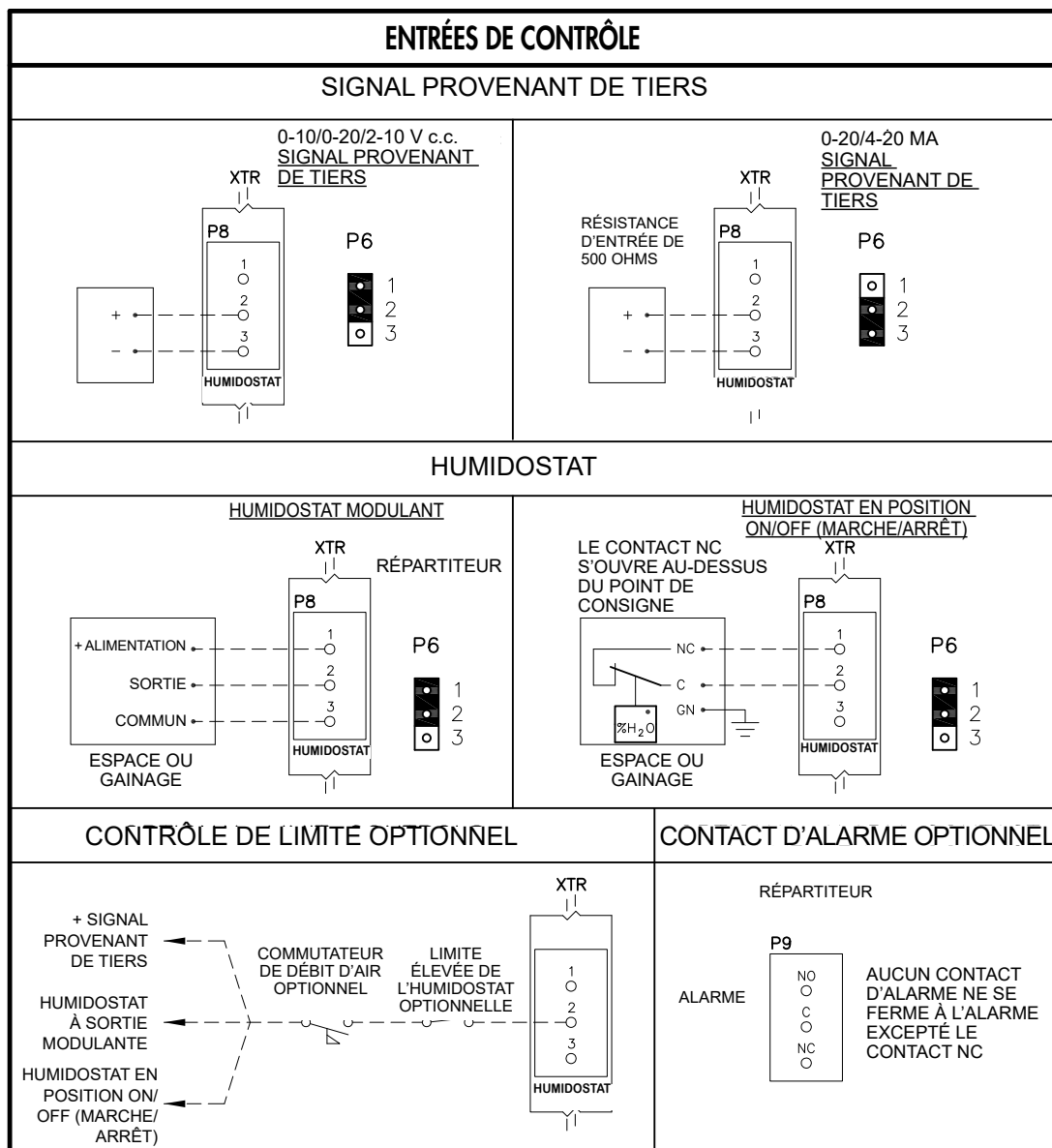
FIGURE 16-1: CONNEXIONS DE CONTRÔLE EXTERNE XTR
