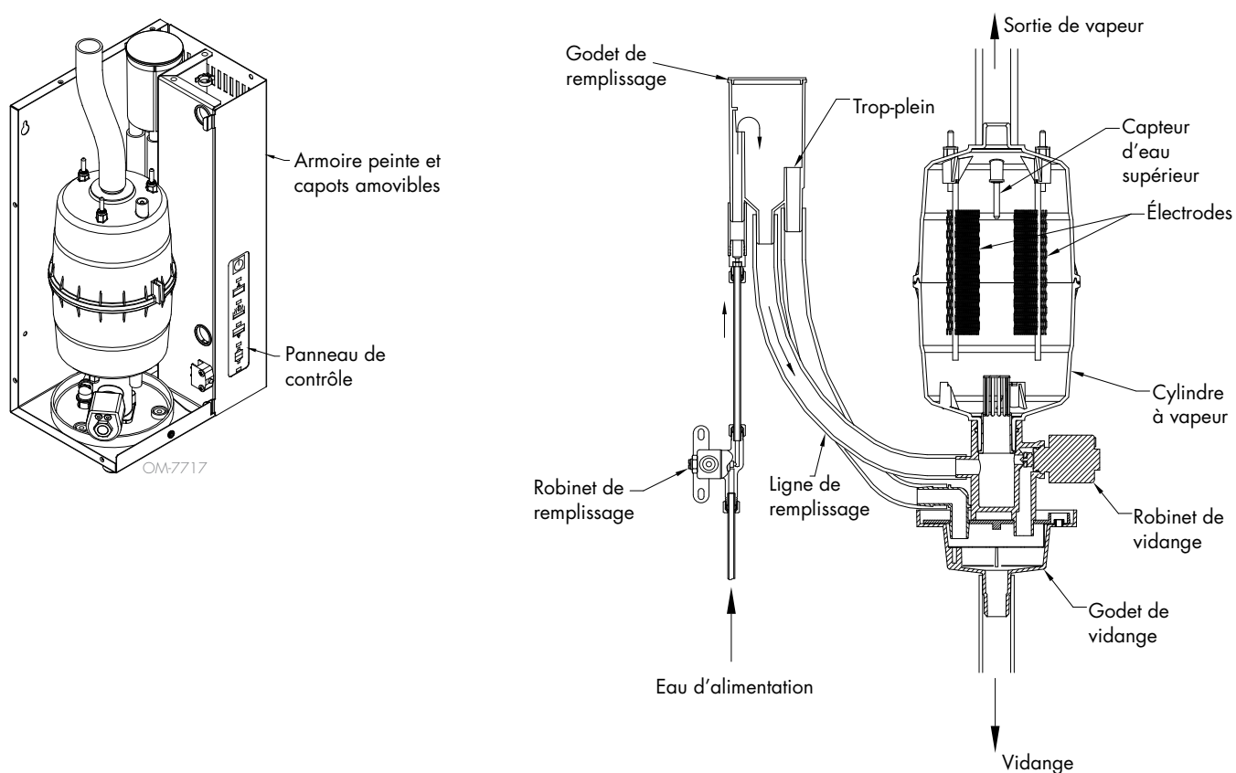
FIGURE 2-1 : COMPOSANTS DE L'HUMIDIFICATEUR XTR
