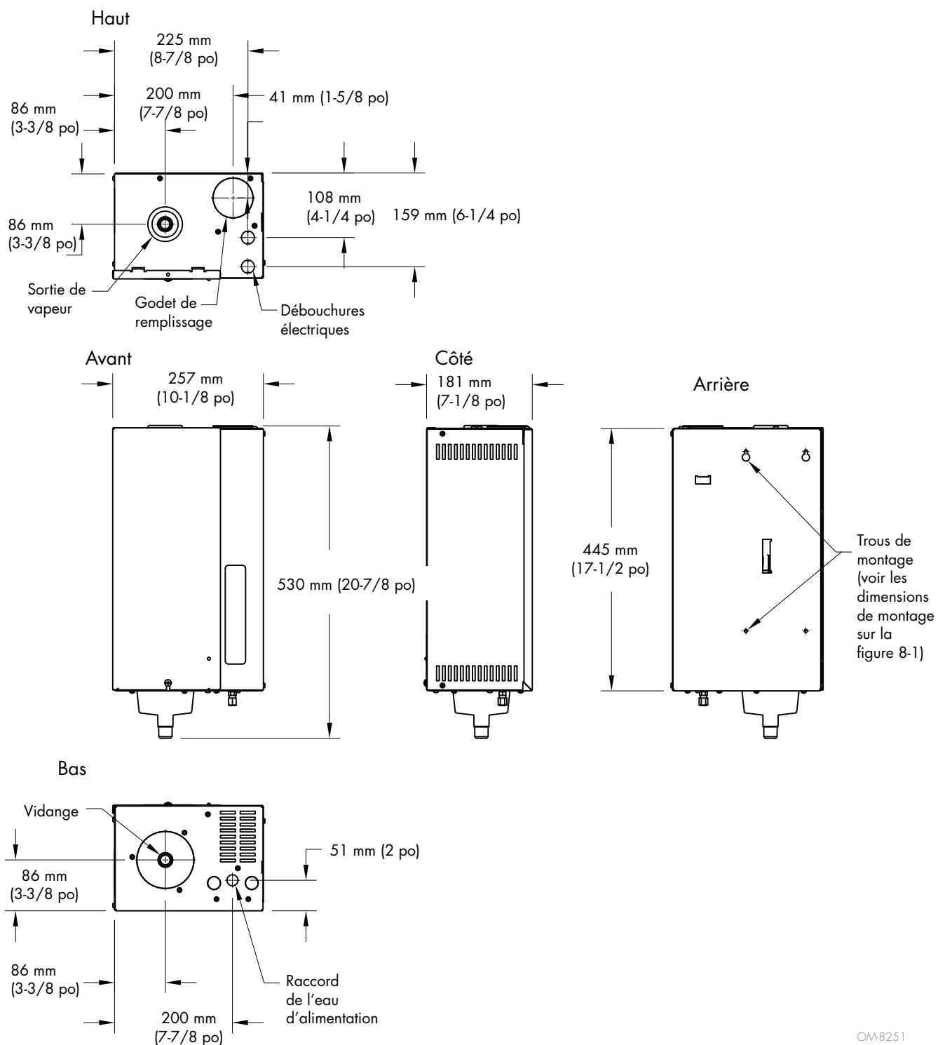
FIGURE 4-1 : DIMENSIONS DE L'HUMIDIFICATEUR XTR
