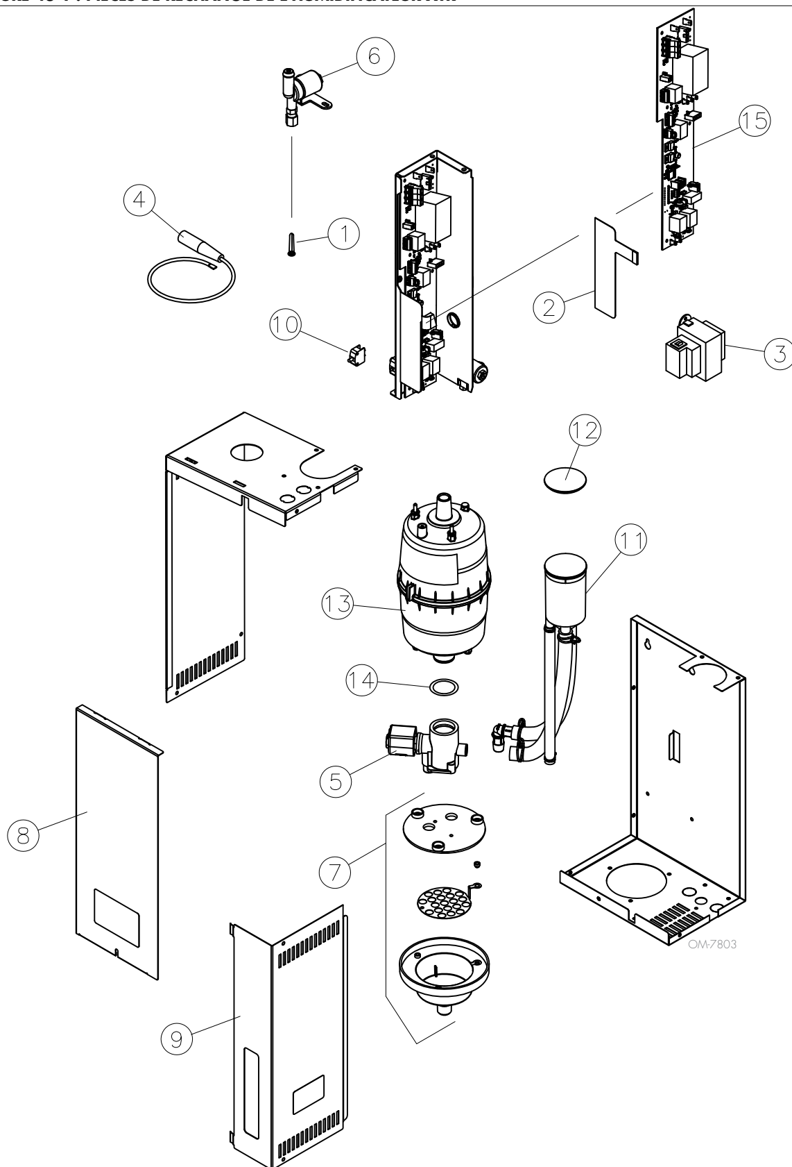
FIGURE 48-1 : PIÈCES DE RECHANGE DE L'HUMIDIFICATEUR XTR
