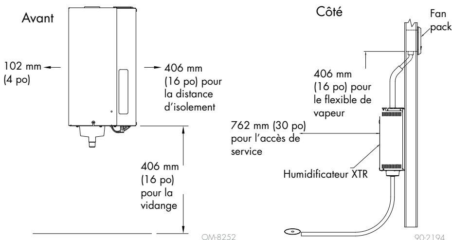
FIGURE 7-1 : DÉGAGEMENTS MINIMUM RECOMMANDÉS POUR LES HUMIDIFICATEURS XTR
