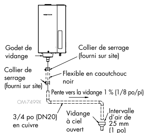
FIGURE 9-1 : DÉTAILS DE LA TUYAUTERIE DE VIDANGE
