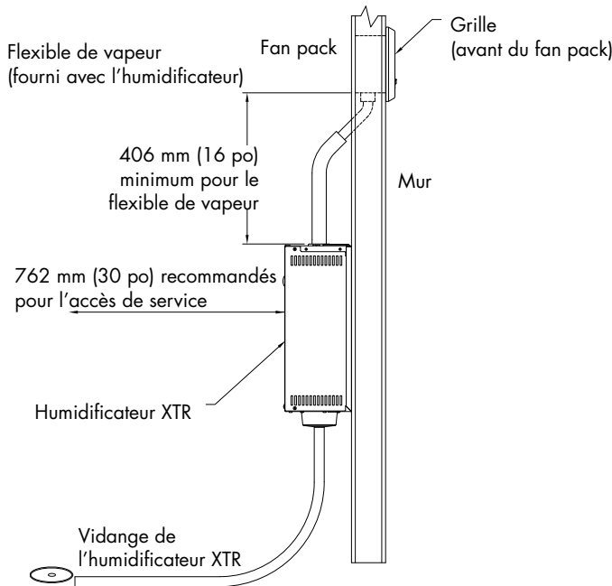
FIGURE 11-2 : RACCORDS À LA TUYAUTERIE DU FAN PACK XTR
